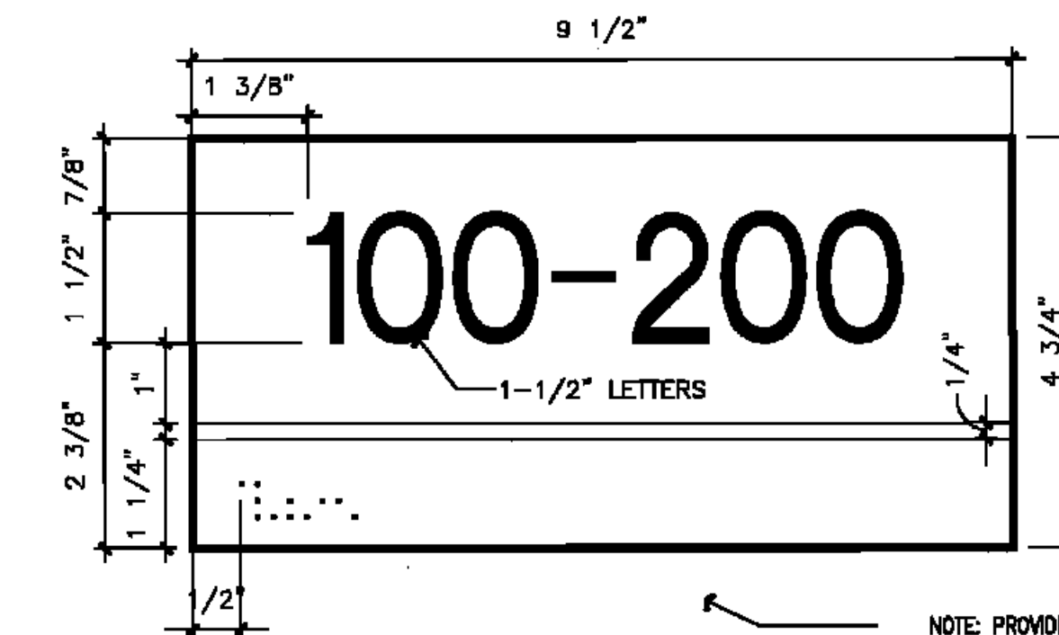
SIGNAGE - TYPE 'G'
