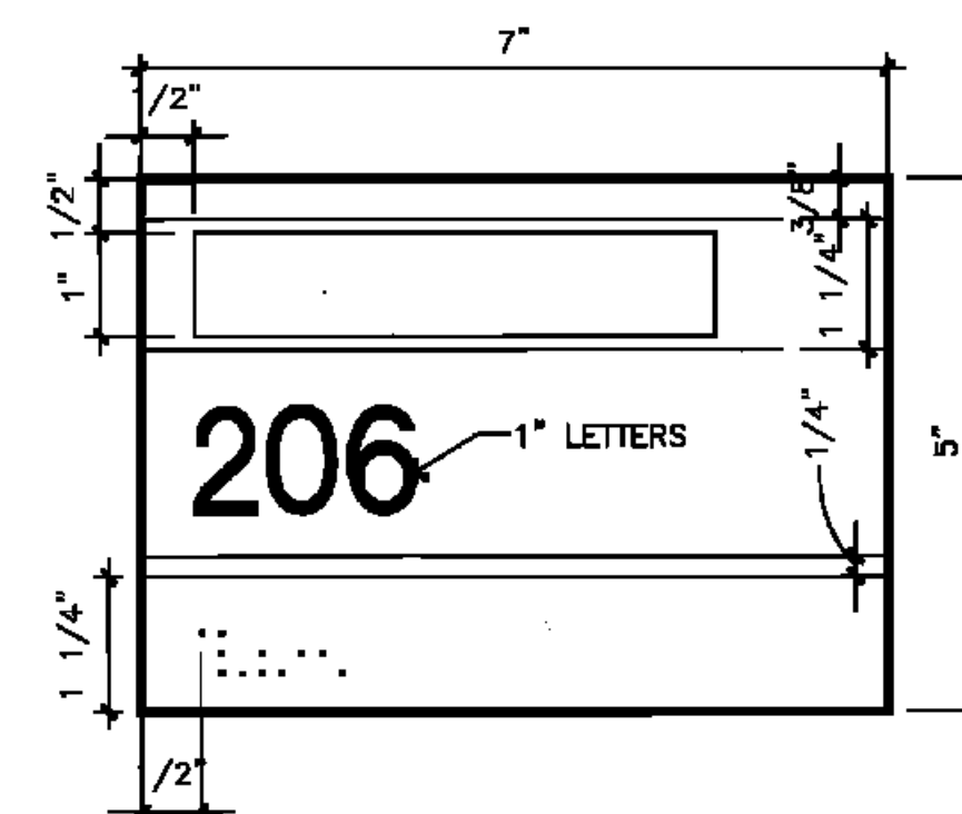
SIGNAGE - TYPE 'B'
